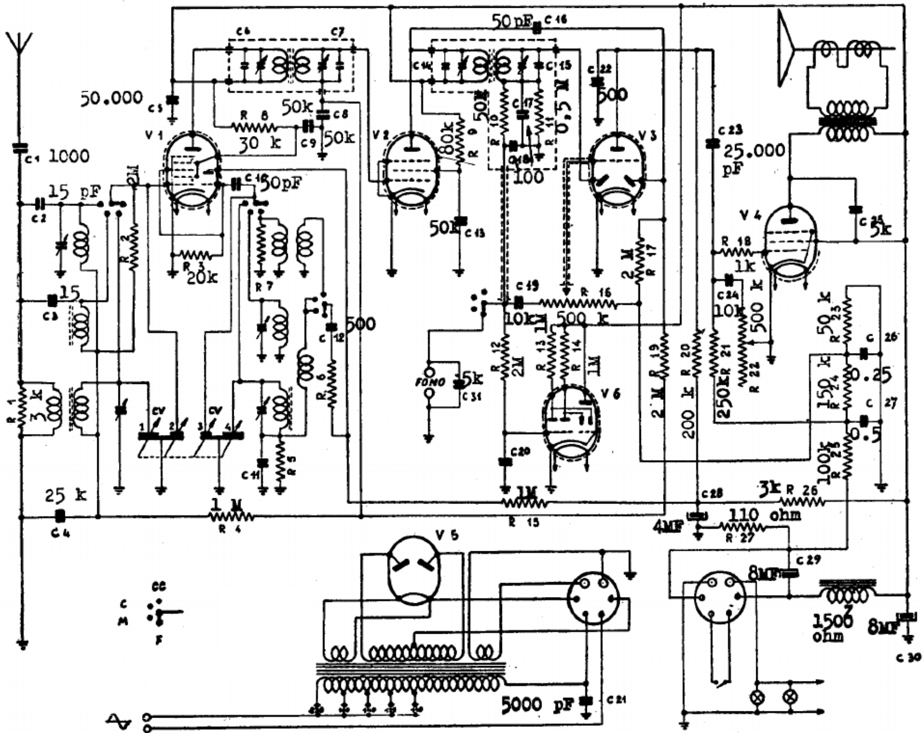
KING'S RADIO Modd. 650 e 680 - VIS RADIO Modd. ADIGE e TEVERE - MF: 465 kc/s. Tensioni: ECH4 pl. 245, sch. 95, osc. 105 gr. - 2,5. EF9 pl. 245, sch. 100, gr. - 2,5. EBC3 pl. 90, gr. - 2,5. EL3 pl. 235, sch. 245, gr. - 5,6 V.
